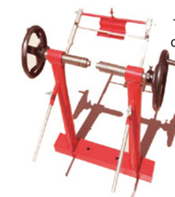
Giá cân vành VGCV0101
