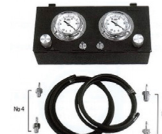
Đo áp suất chân không VT2 TOYO NPA Japan
