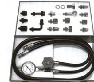
Kiểm tra áp suất dầu trợ lực PS-150 TOYO NPA Japan
