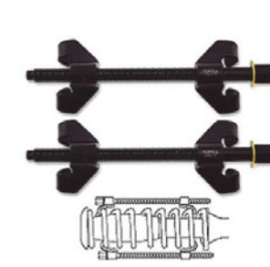
Cảo lò xo JEAC0127
